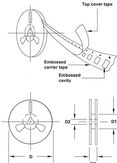
DO-214AB(SMC) - Reel
